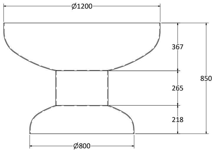
VISTA FRONTALE
